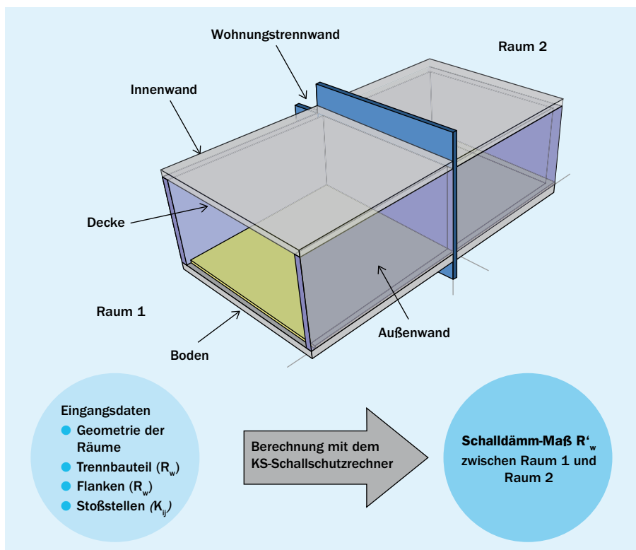
Von der Bauteileigenschaft R_w zur Gebäudeeigenschaft R'_w
