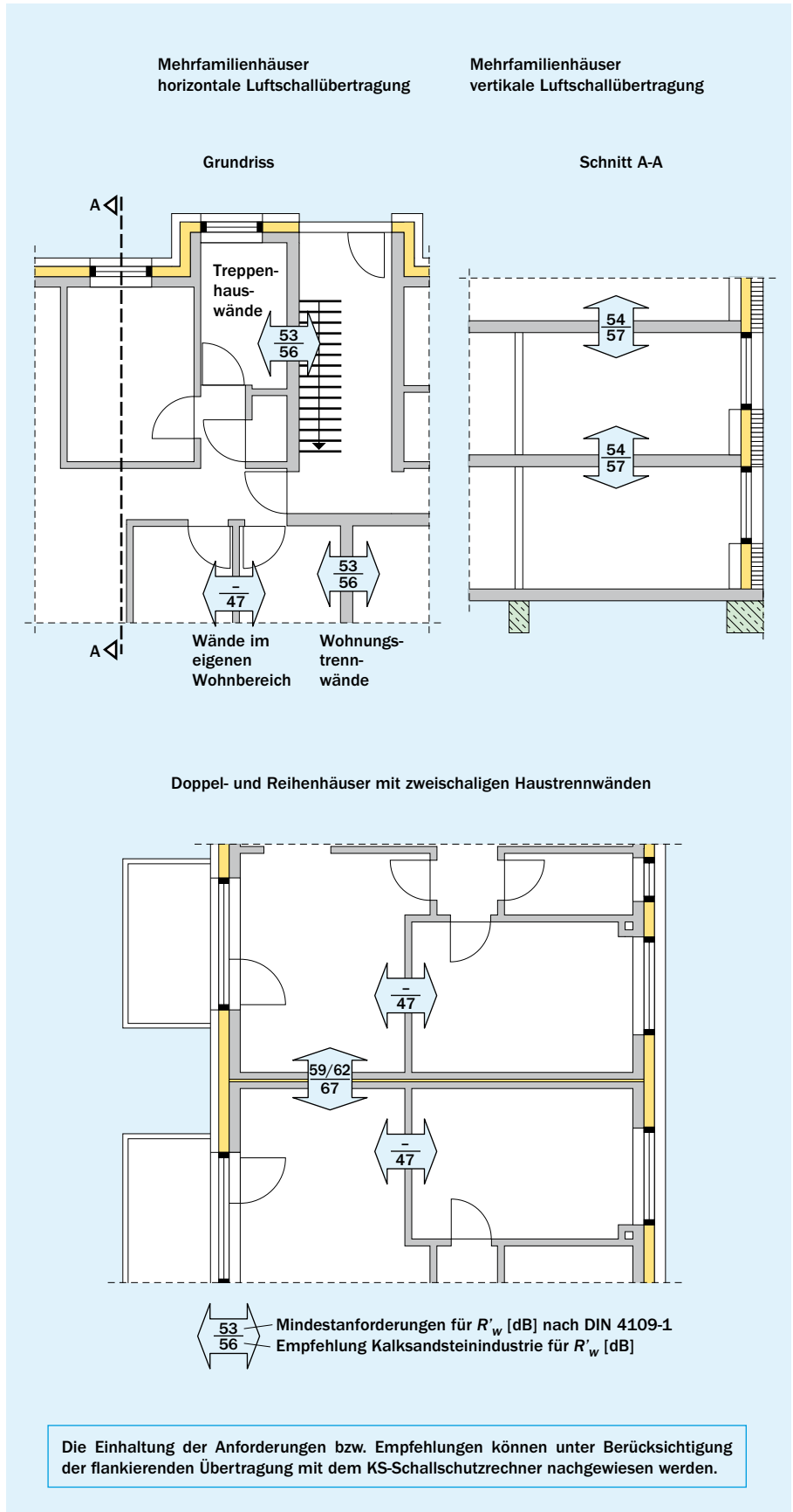
Mindestanforderungen nach DIN 4109-1 und Empfehlungen der Kalksandsteinindustrie für die erhöhte Luftschalldämmung ( R'_w )
