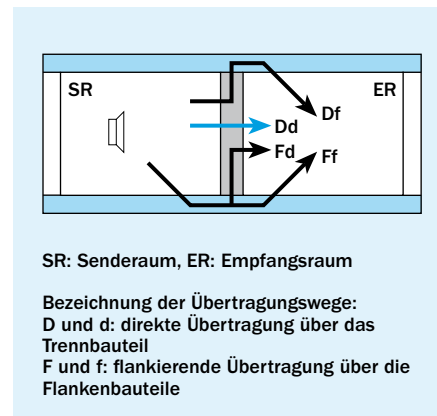
Direkte und flankierende Übertragungswerte zwischen zwei Räumen
