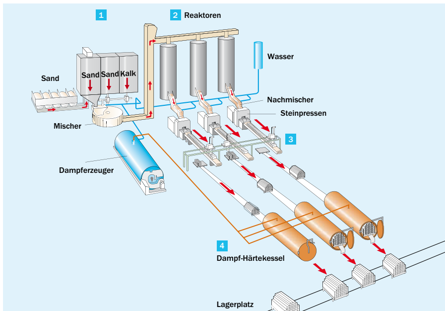
Herstellung von Kalksandstein
