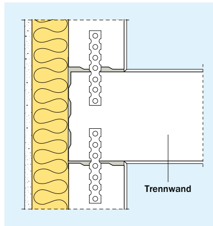
Trennwand durchgeführt, flankierende Wände stumpf angeschlossen
